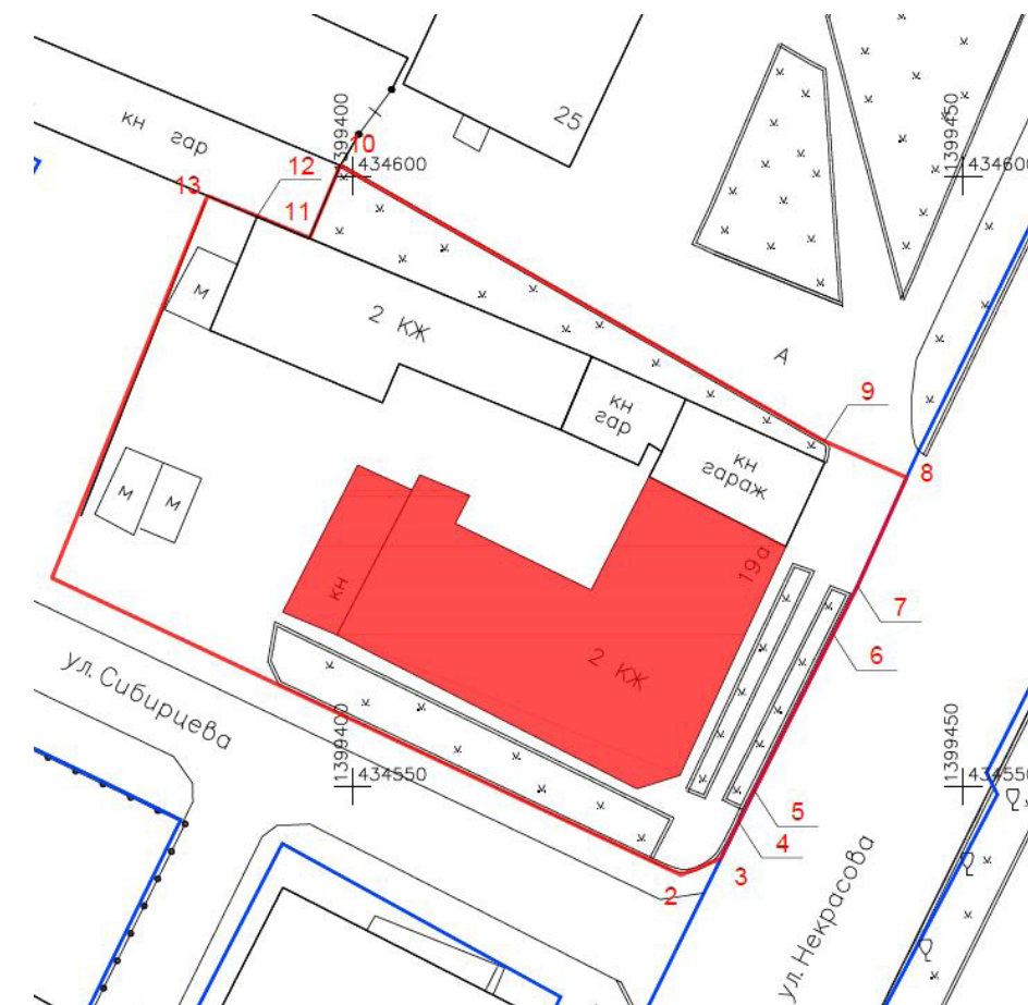
2. Объемно-пространственная композиция
